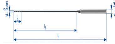
cod 50780 - 80xD
